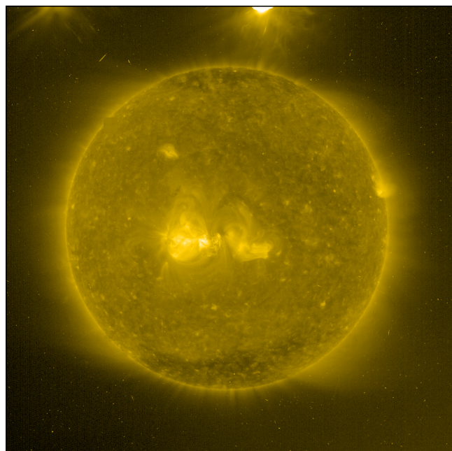
Fe XV 284 A
