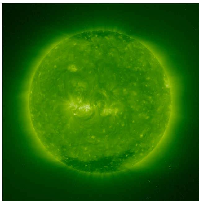
Fe XII 195 A
